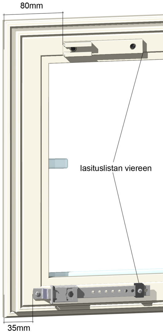
Sisäpuite
